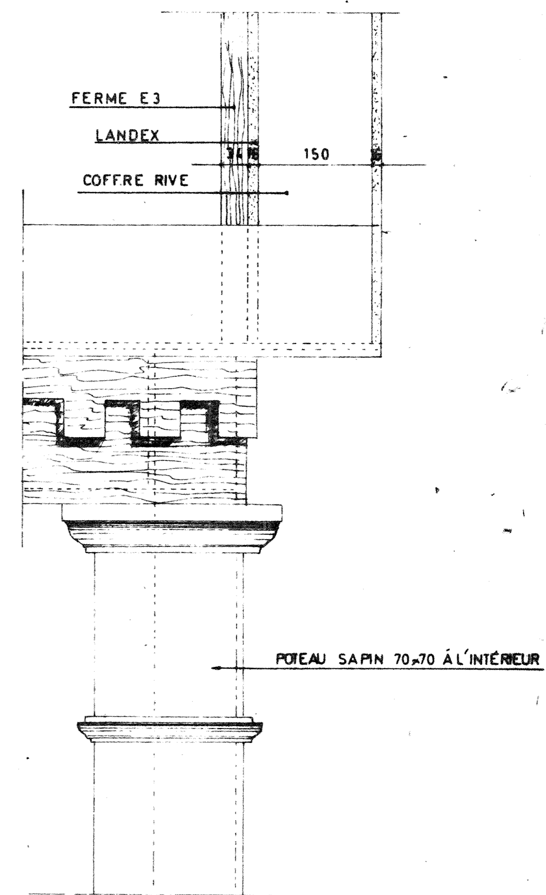
POTEAU D'ANGLE VUE DE LA FAÇADE PRINCIPALE
