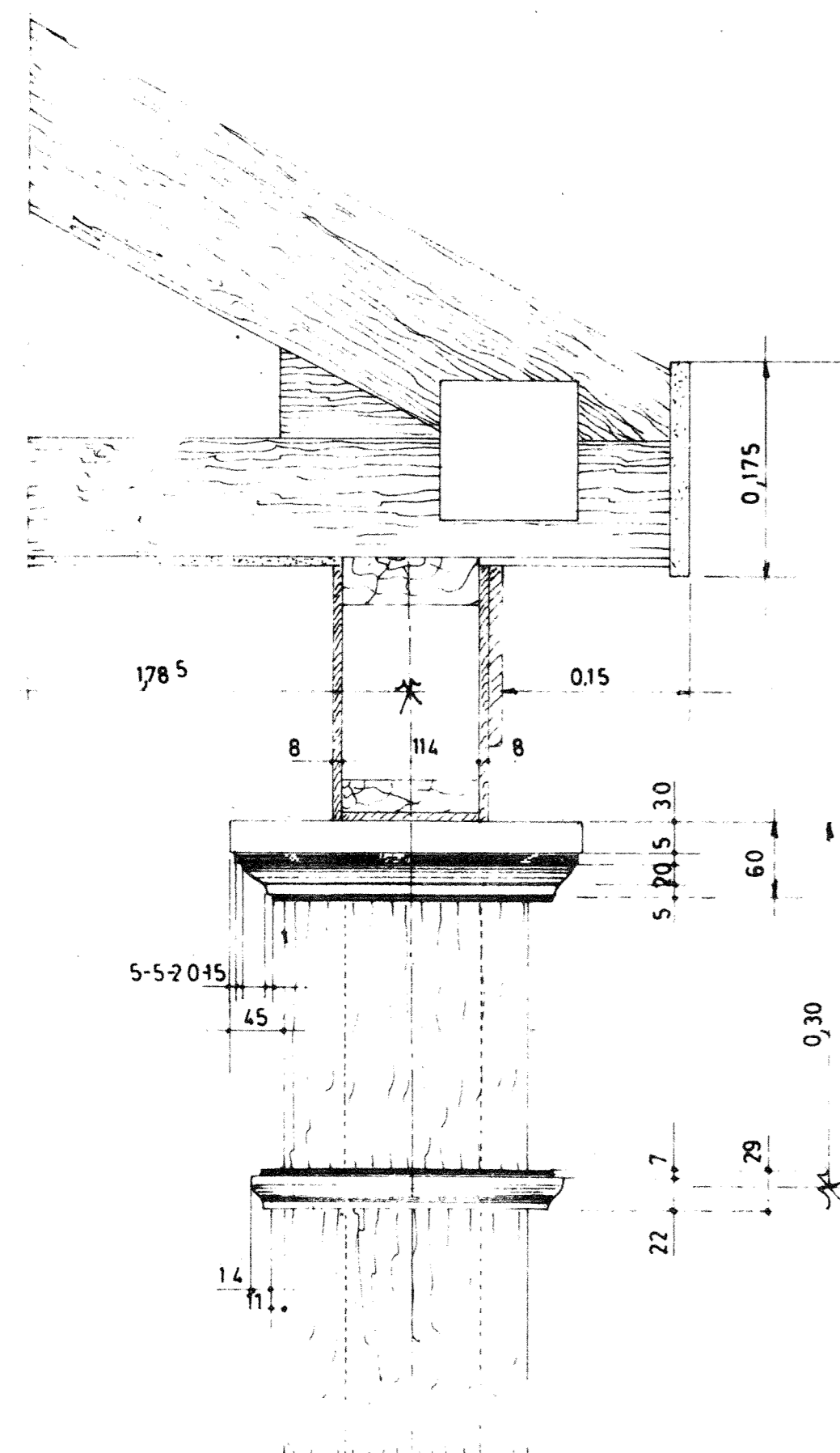
COUPE A-B
